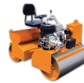
AB-308 테니스장 전동롤러 · \phi 500×900, \phi 500×1200
