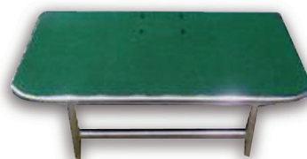
AS-4003 스타트대 받침대 / 경기용 · 800×1200×300mm
