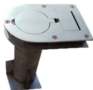
AB-2002 배구금구 / 실내용, 스텐 · 후로링용, 250mm, 200mm, 150mm · 상판 145×220mm
