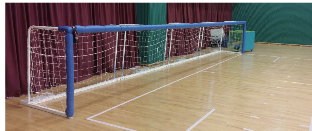
AB-706 골볼골대 / 보호대포함 · 4단 분리형으로 제작 · 정전기 분체도장 · 흔들림 방지 무게판 사용제작
