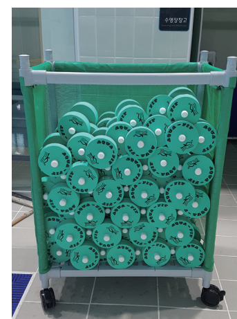
AS-36 덤벨보관함 / P.V.C · 870×510×1330mm(L×W×H)
