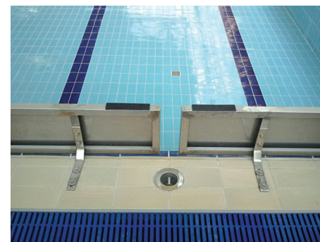
AS-230 터치판걸이 · 2400×300mm(L×H)
