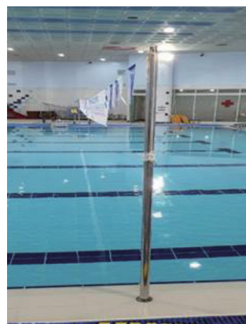
AS-81 배영턴표시 지주 · H : 2000mm
